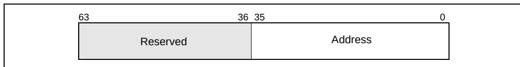
Figure 13-7. IA32_MCi_ADDR MSR
